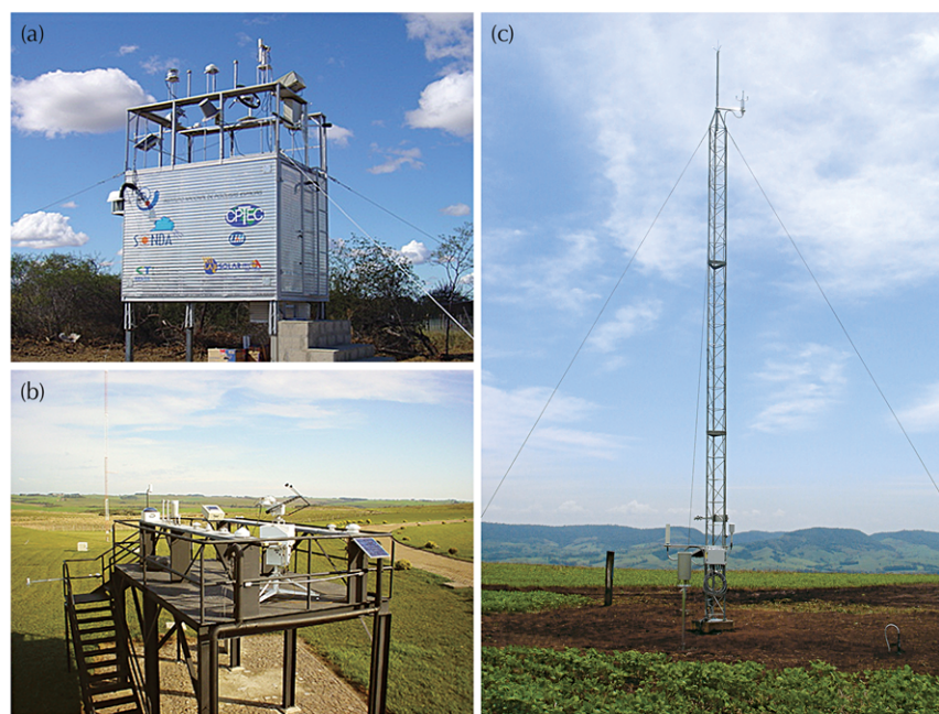
Figura 11. (a) Módulo de medidas da estação SONDA em Brasília com os sensores de radiação instalados sobre o teto; (b) Plataforma com os sensores de radiação na estação SONDA em São Martinho da Serra; e (c) Plataforma de coleta de dados
