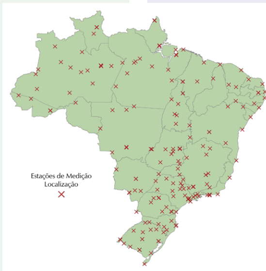
Figura 5. Localização das estações da base de dados do NCDC.
