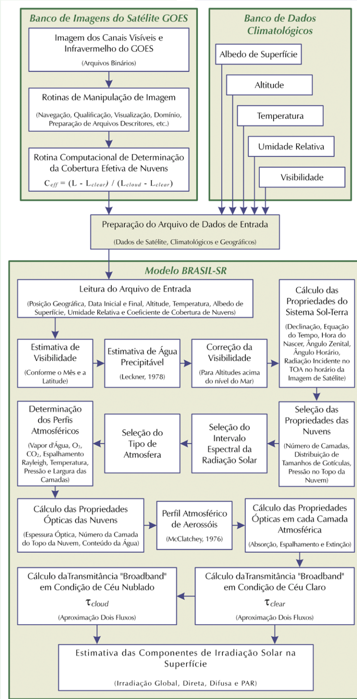
Figura 4. Fluxograma do modelo de transferência radiativa BRASIL-SR.
